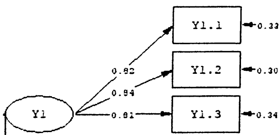
Gambar 14 Model Pengukuran variabel laten pengembangan SDM perhotelan.
