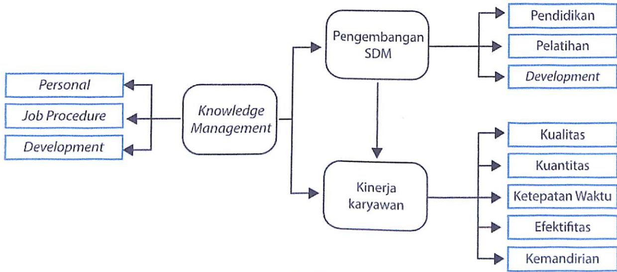
Gambar 2 Struktur analisis variabel penelitian
