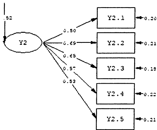
Gambar 15 Model Pengukuran variabel laten kinerja karyawan hotel
